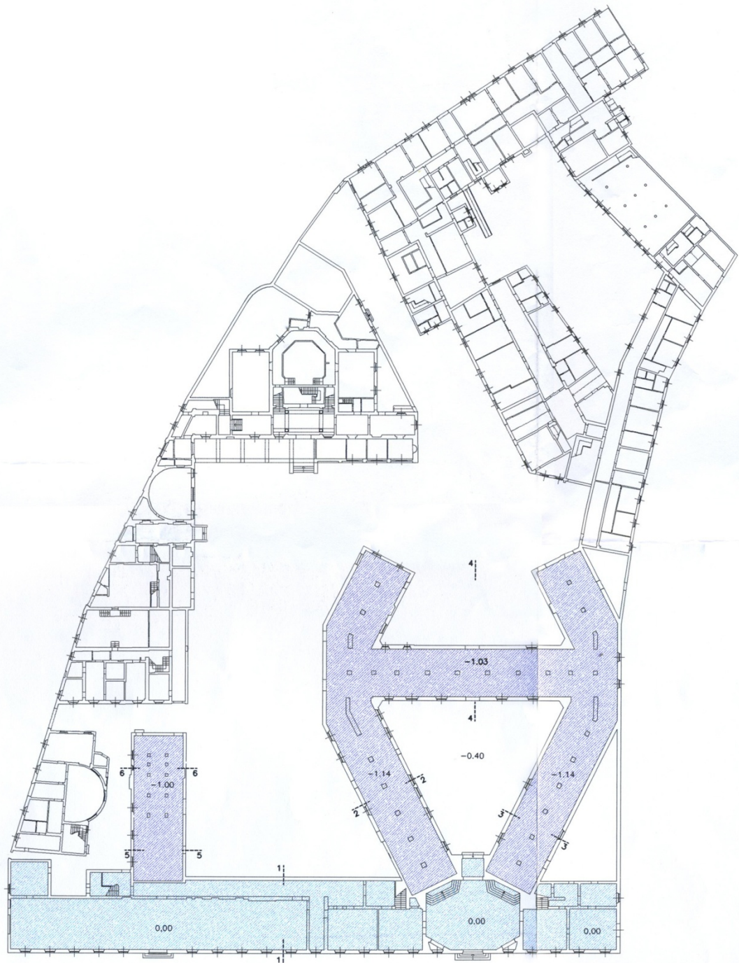
PIANTA DA QUOTA -1,14, A QUOTA 0,00
